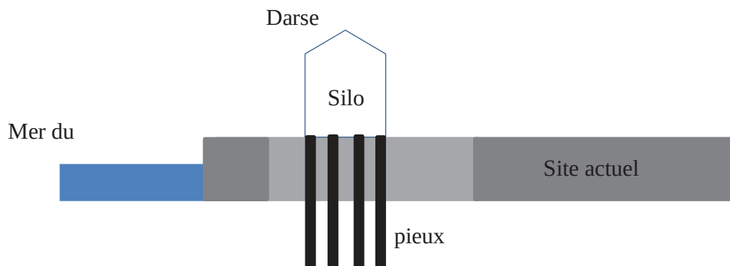
Schéma de principe fondations spéciales de profondeur supérieure à la zone comblée
